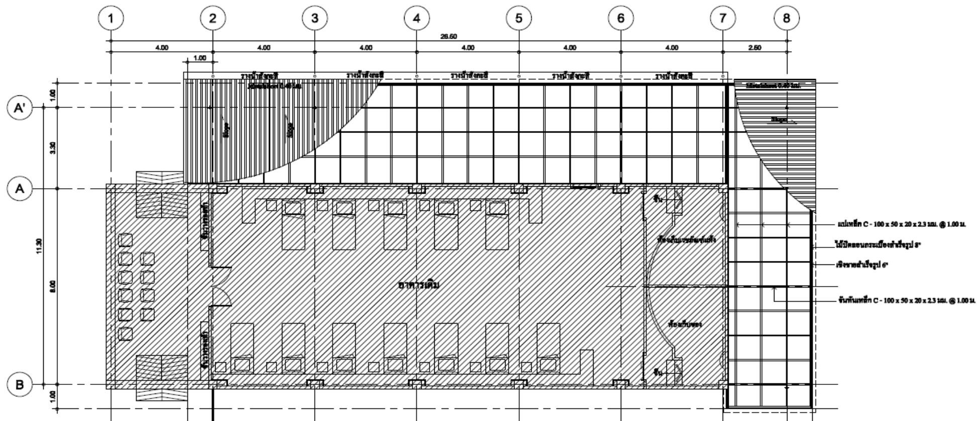
แปลนโครงสร้างหลังคา มาตราส่วน 1:100
